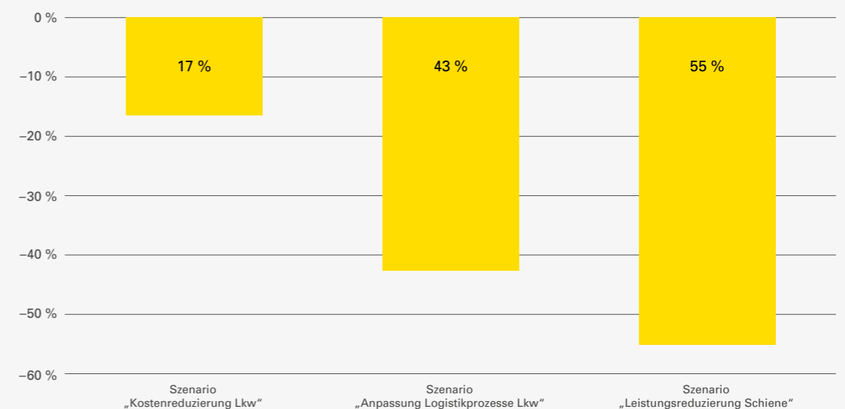
Abbildung 3.10: Relativer Rückgang der Verkehrsleistung des Schienengüterverkehrs unter den drei Umsetzungsszenarien des automatisierten Straßengüterverkehrs für das Jahr 2035 im Vergleich zu 2010
